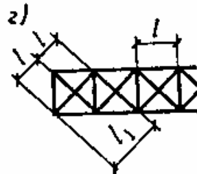
Черт. 6. Схемы решеток ферм для определения расчетной длины элементов
